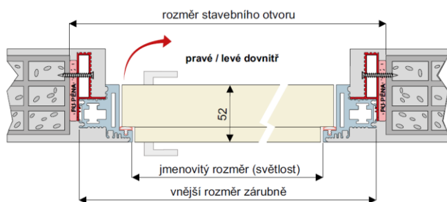
FORTIUS 52 zárubeň pro zdivo, otvírání dovnitř – reverzní
