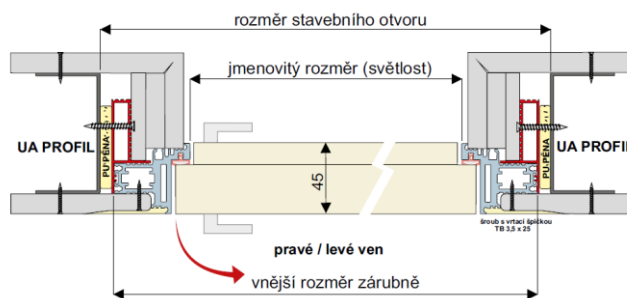
DURUS 45 zárubeň pro SDK, jednoduché opláštění, otvírání ven
